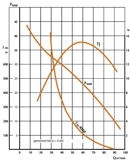
Druckluft-Sparlüfter; Type SL 4
