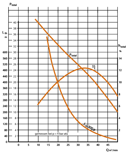
Druckluft-Sparlüfter; Type SL 3
